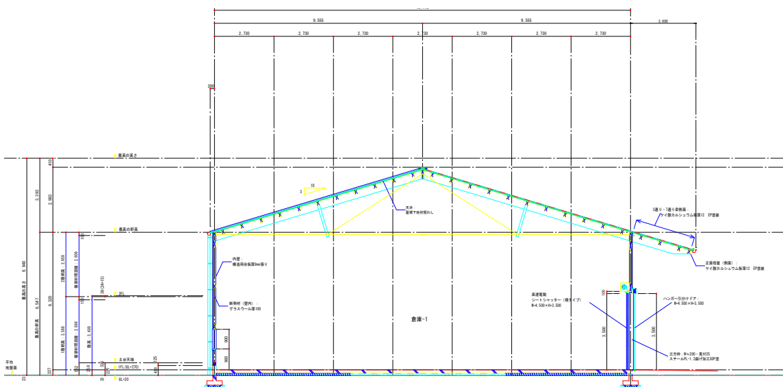
断面図1（北東妻側）
